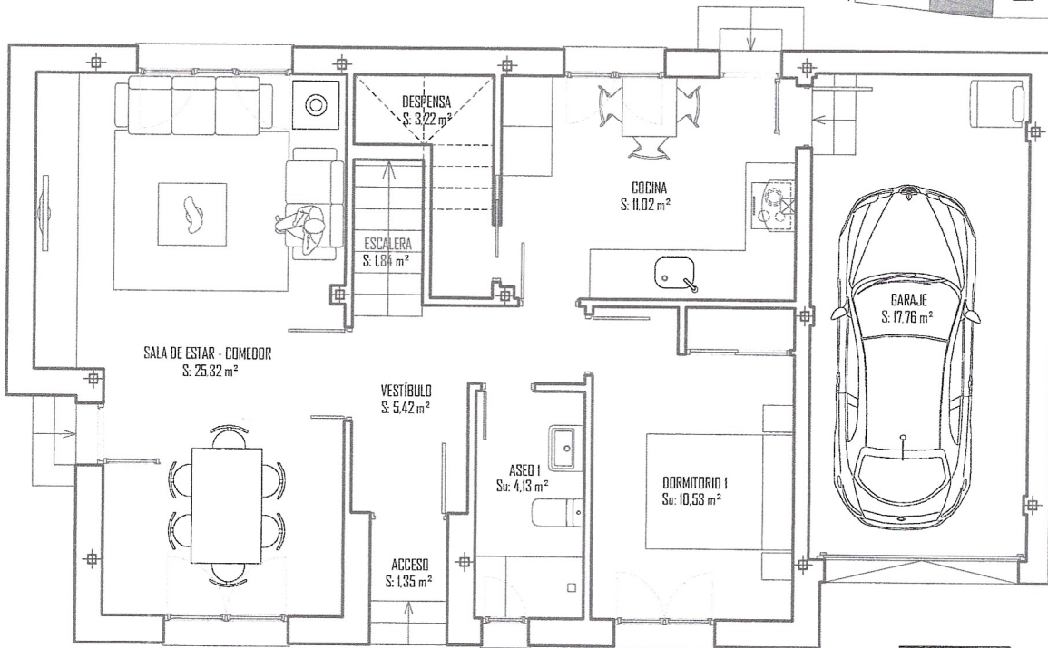
PLANTA BAJA
